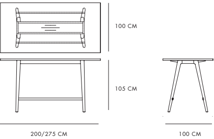
STEHTISCH 1510/STANDING TABLE 1510
